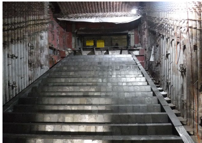
2号焼却炉 耐火物(施工中)
