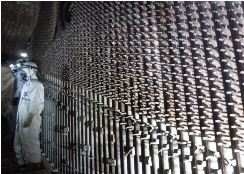
2号ボイラー(施工前)
